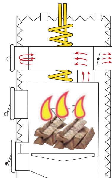
Vedeldstads genomskärning
